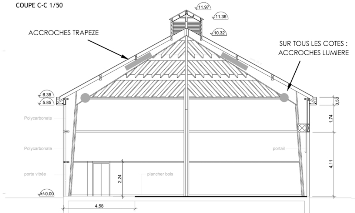
COUPE C-C 1/50
